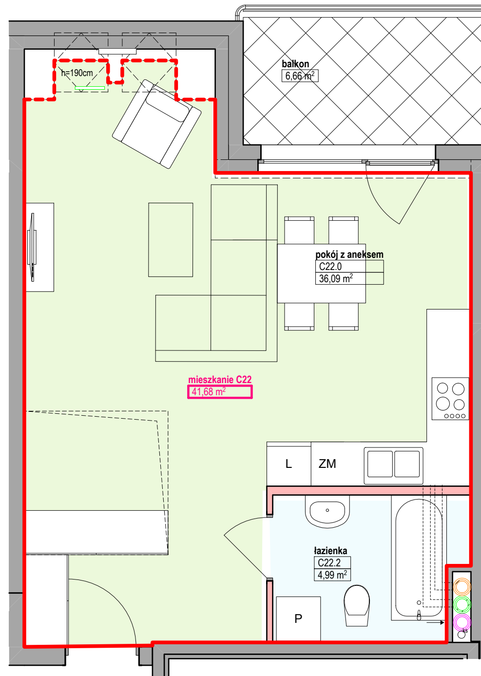
KONDYGNACJA 1
