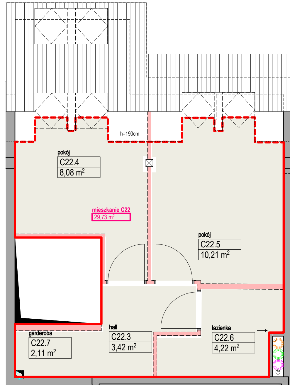
KONDYGNACJA 2
